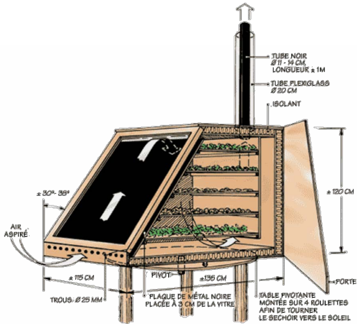
Exemple de séchoir solaire
